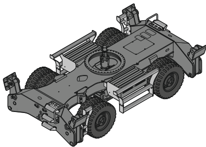
Pneus e quatro patolas
