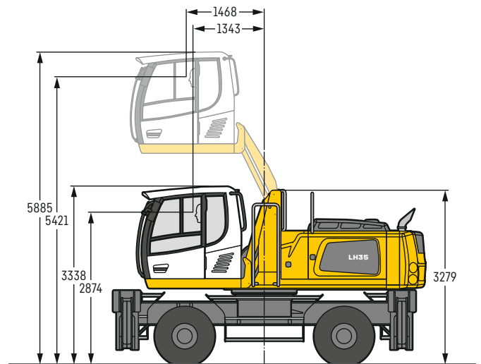
Rehausse de cabine LHC 255 (rehausse hydraulique)
